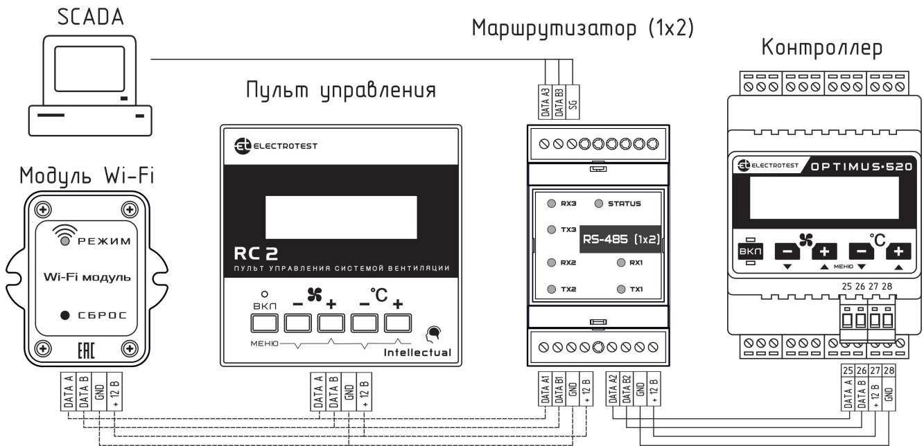
Рис. 2.3 Подключение средств ДУ + SCADA
