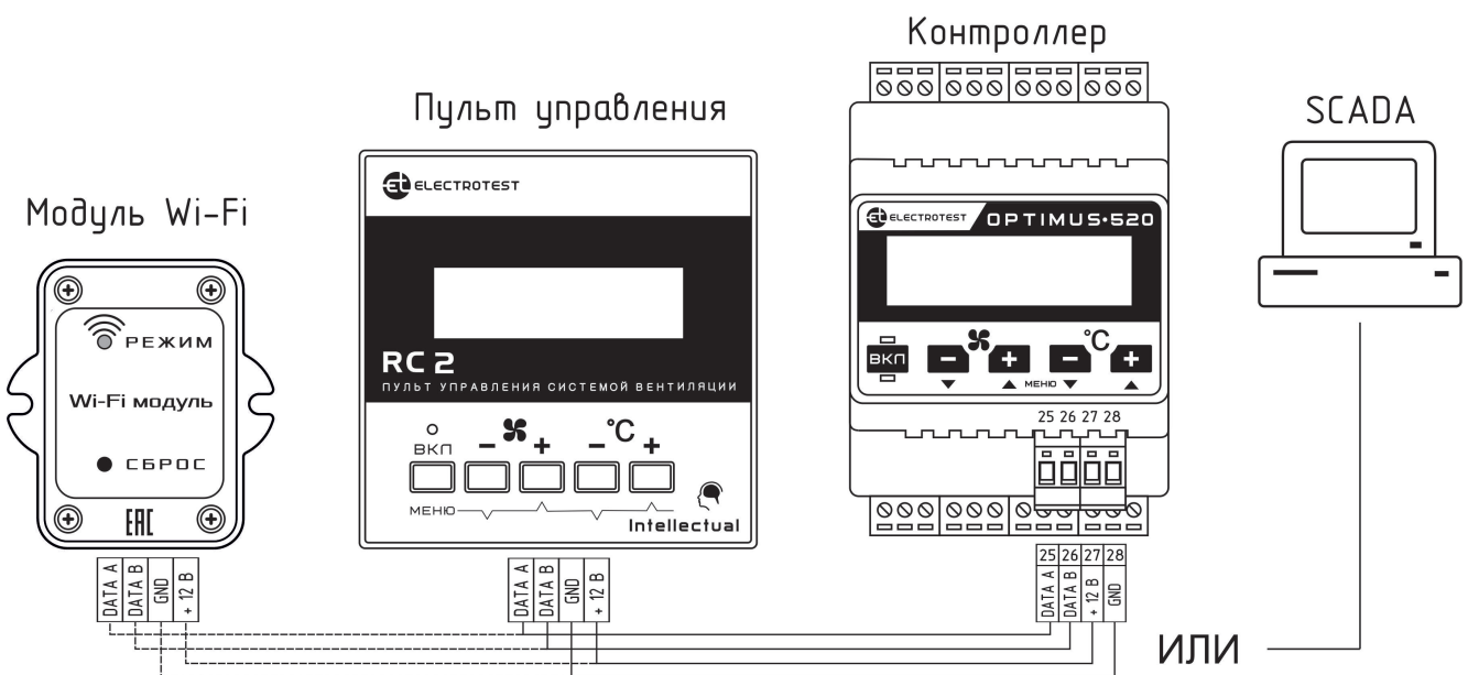
Рис. 2.2 Подключение средств ДУ
