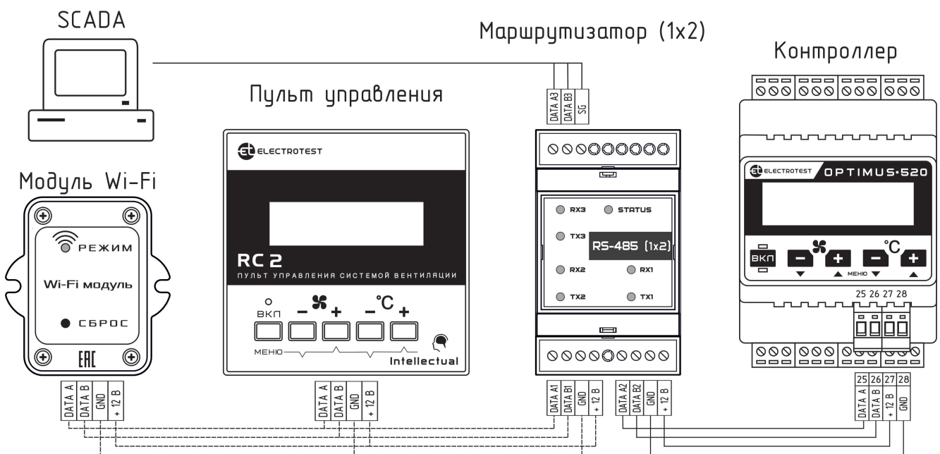
Рис. 6.4 Подключение внешних средств ДУ + SCADA
